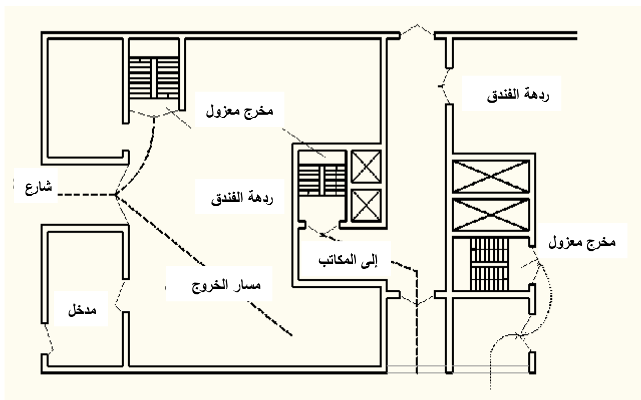
الشكل 4-5: مثال على مكونات وسيلة الخروج
