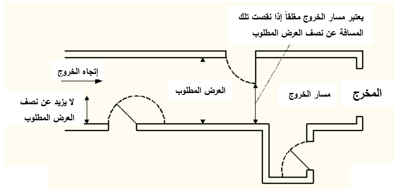
الشكل 4-2/3: الأبواب التي تكون زاوية فتحتها 180 درجة
