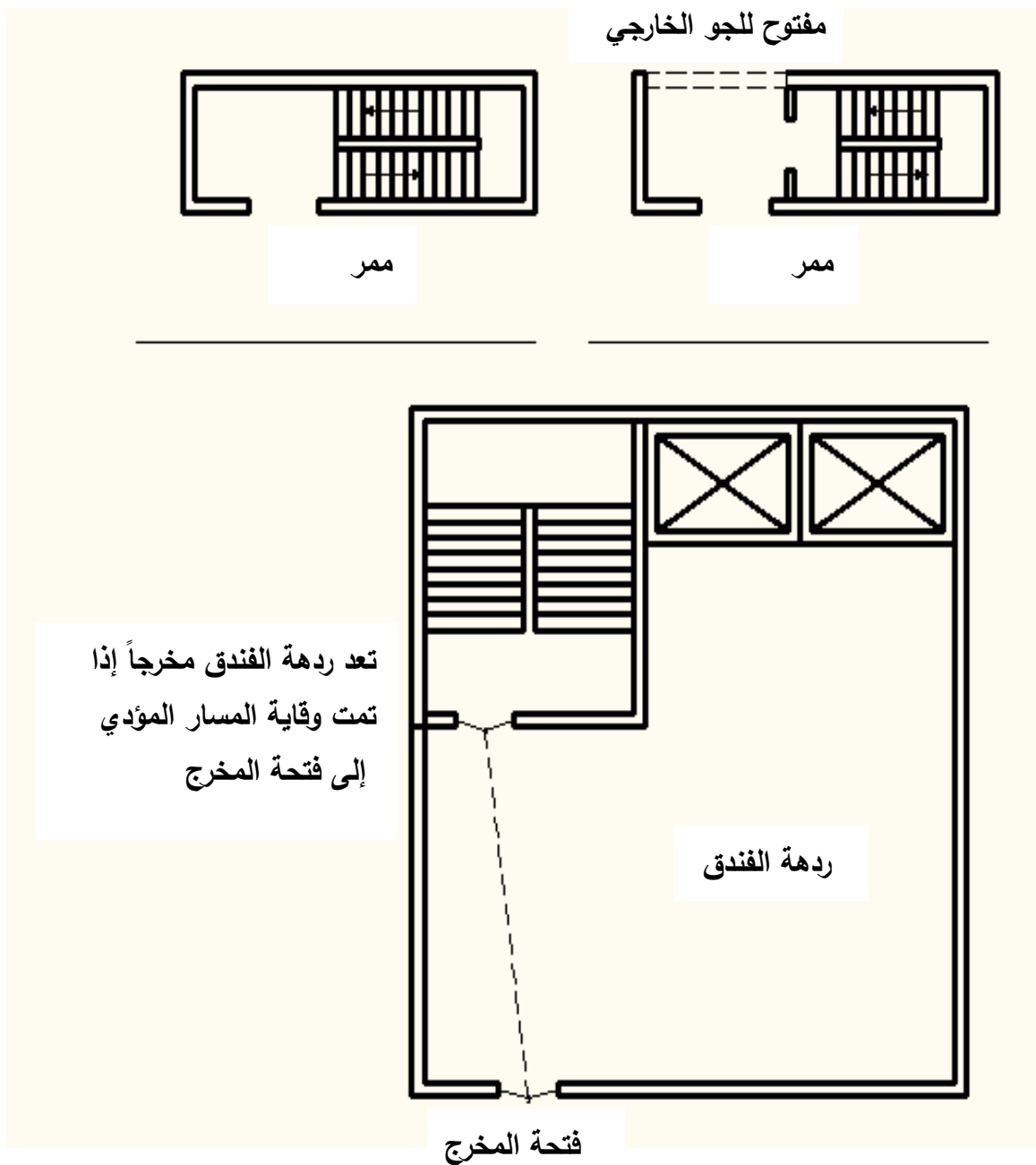
الشكل 4-3/1: أنواع مختلفة من المخارج
