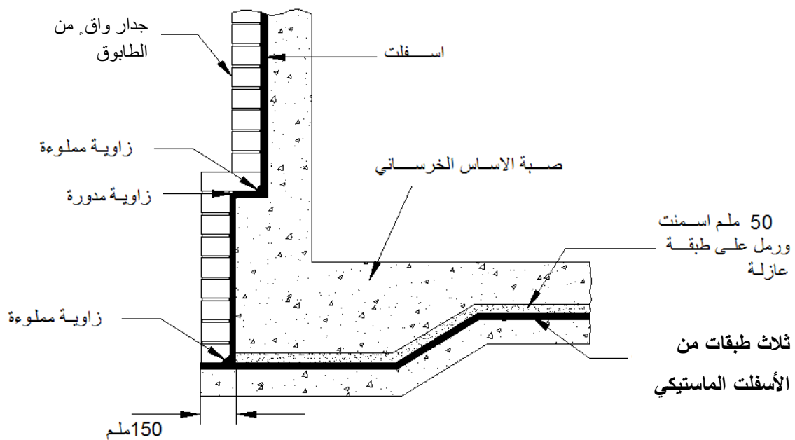
الشكل 3/7-5: مثال تطبيقي لتنفيذ الحماية الحوضية بالاسفلت الماستيكي من الخارج
