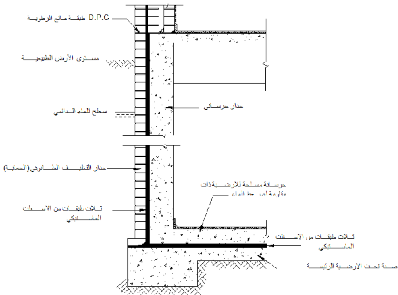
الشكل 8-1/3: عزل السرايب ضد تأثير المياه الخارجية بوضع الأسفلت الماسطي على الجدار الخرساني من الخارج
