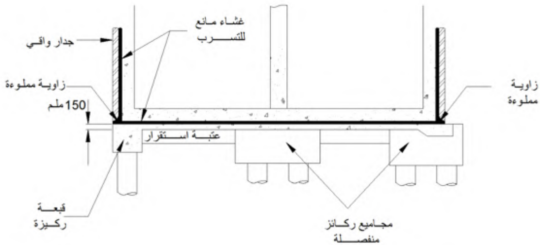
الشكل 5-1/7: طبقة سرداب محمي بالطريقة الحوضية محمول على قبة ركائز
