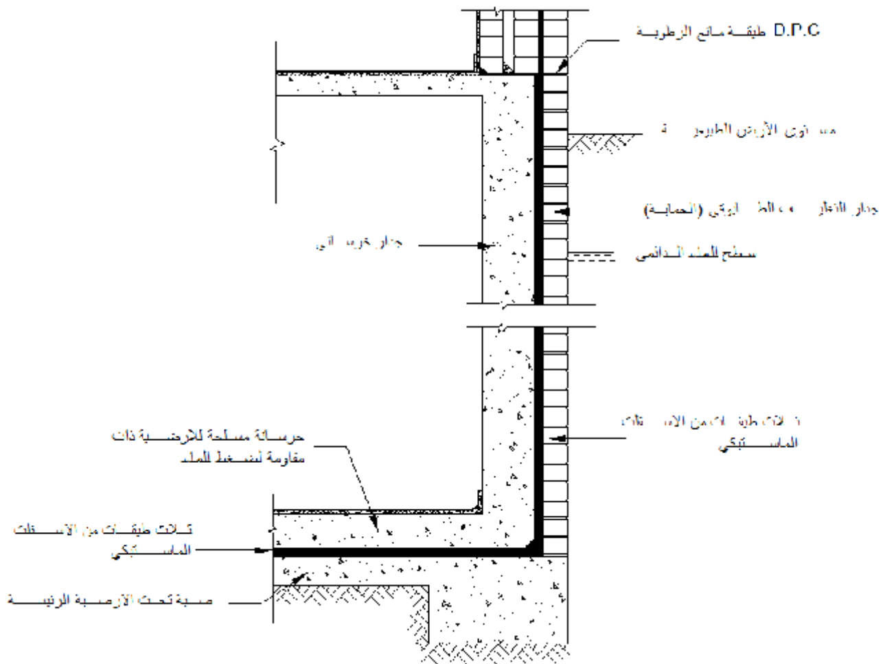
الشكل 8-2/3: عزل السرايب ضد تأثير المياه الخارجية بوضع الأسفلت الماسطي على جدار التغليف من الداخل
