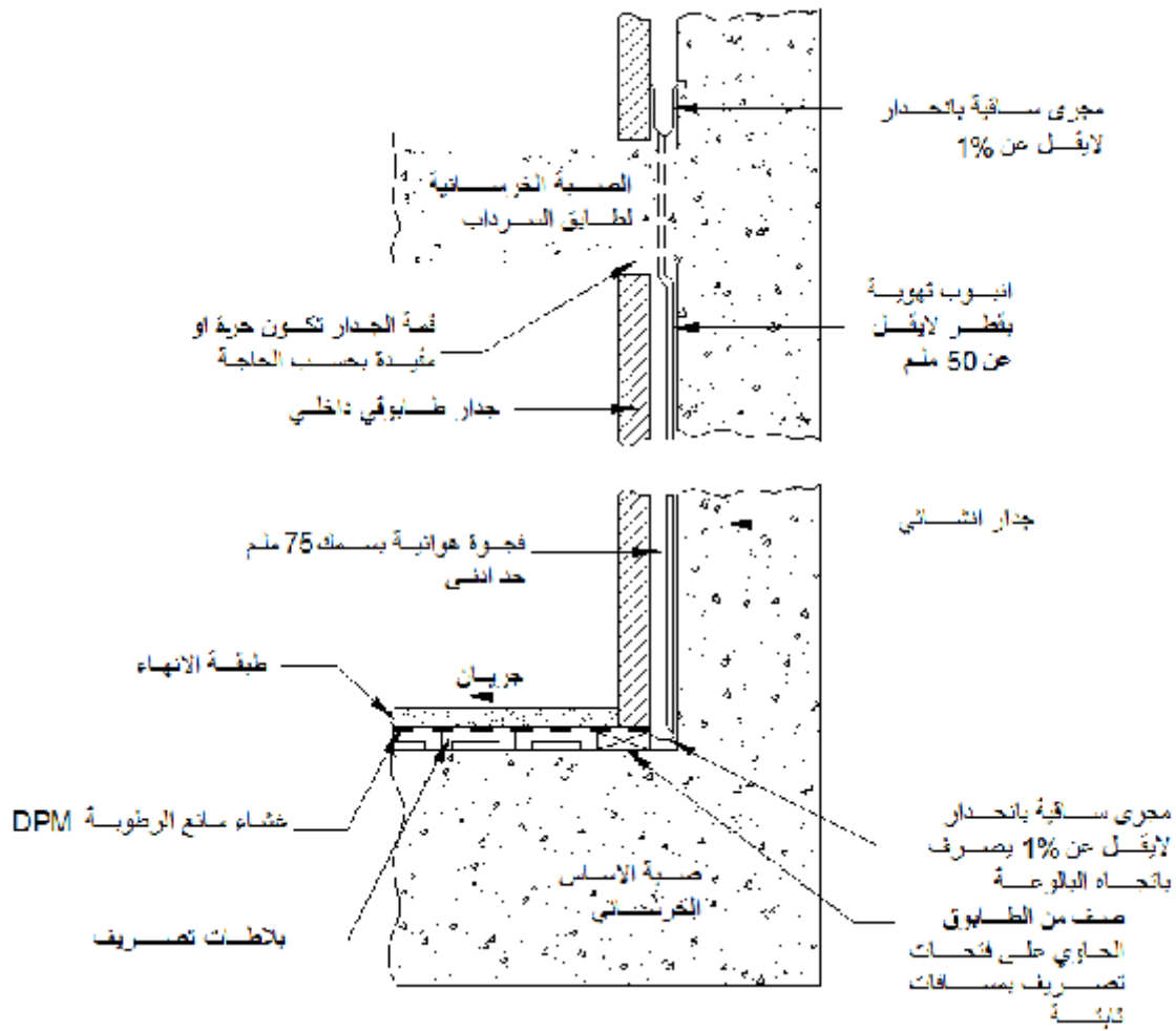
الشكل 4/2-5: مثال تطبيقي لمنشأ يحتوي على فجوات تصريف
