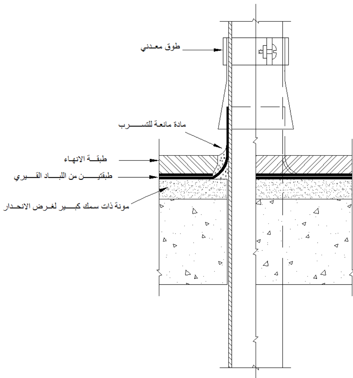
الشكل 8-14/3: تفاصيل معالجة تقاطع انبوب خلال سقف بأستعمال اللباد القيري
