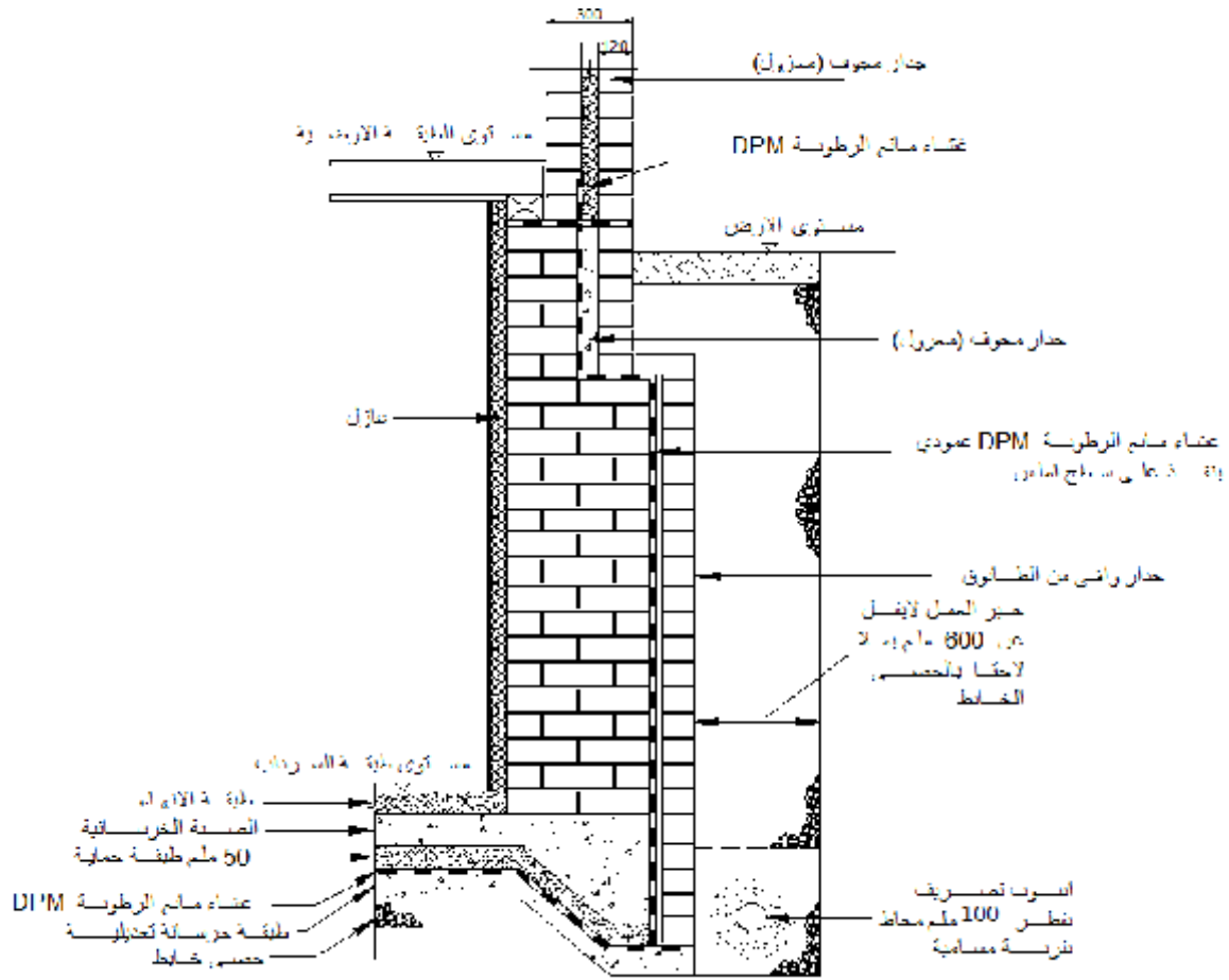
الشكل 5-2/3: مثال تطبيقي لجدار مشيد من مواد البناء غير الخرسانية لا يحتوي على فجوات تصريف
