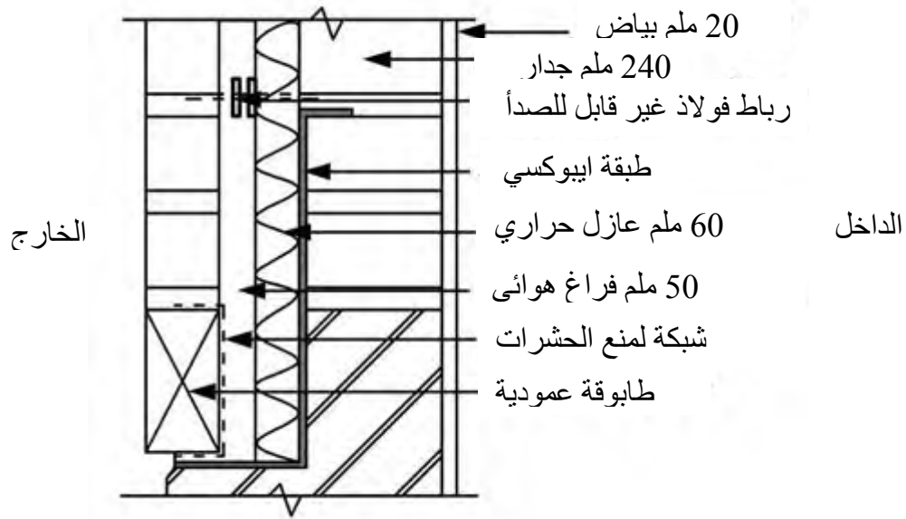
الشكل 4-7: نموذج جدار لتثبيت عازل حراري يتأثر بالرطوبة (الابعاد هي للمثال) (يثبت معيق البخار بحسب الفقرة 5/4/8-7)
