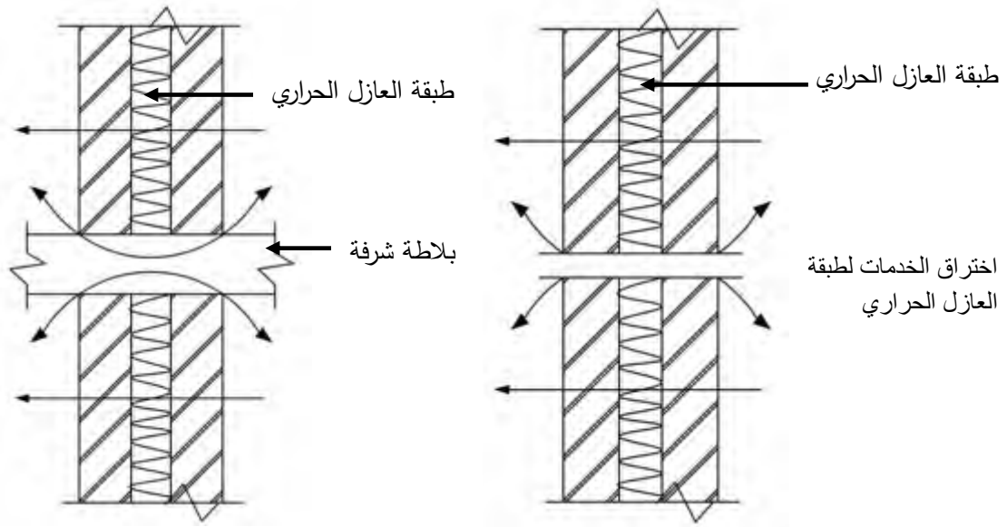
أ- اختراق بعض الخدمات (مثل انابيب المياه، مجاري الهواء وغيرها) طبقة العازل ب- تقاطع الجدار مع بلاطة شرفة الشكل 4-1: أمثلة لبعض احتمالات الجسور الحرارية الانشائية
