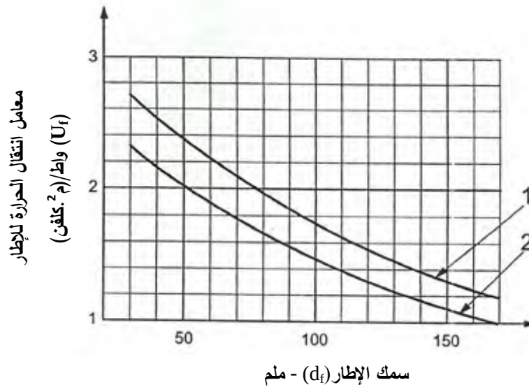
الشكل 5/5-4: معامل انتقال الحرارة الاجمالي للأطر الخشبية وأطر الخشب-المعدن بالاعتماد على سمك الإطار، d_f ، لاحظ الشكل 6/5-4 [4].
