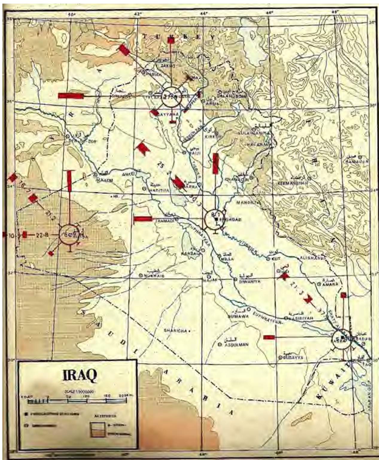
الشكل 2-11: المعدل الشهري لتكرارات الرياح "سرعة واتجاهاً" ضمن الاتجاهات المعينة خلال شهر تموز [2]
