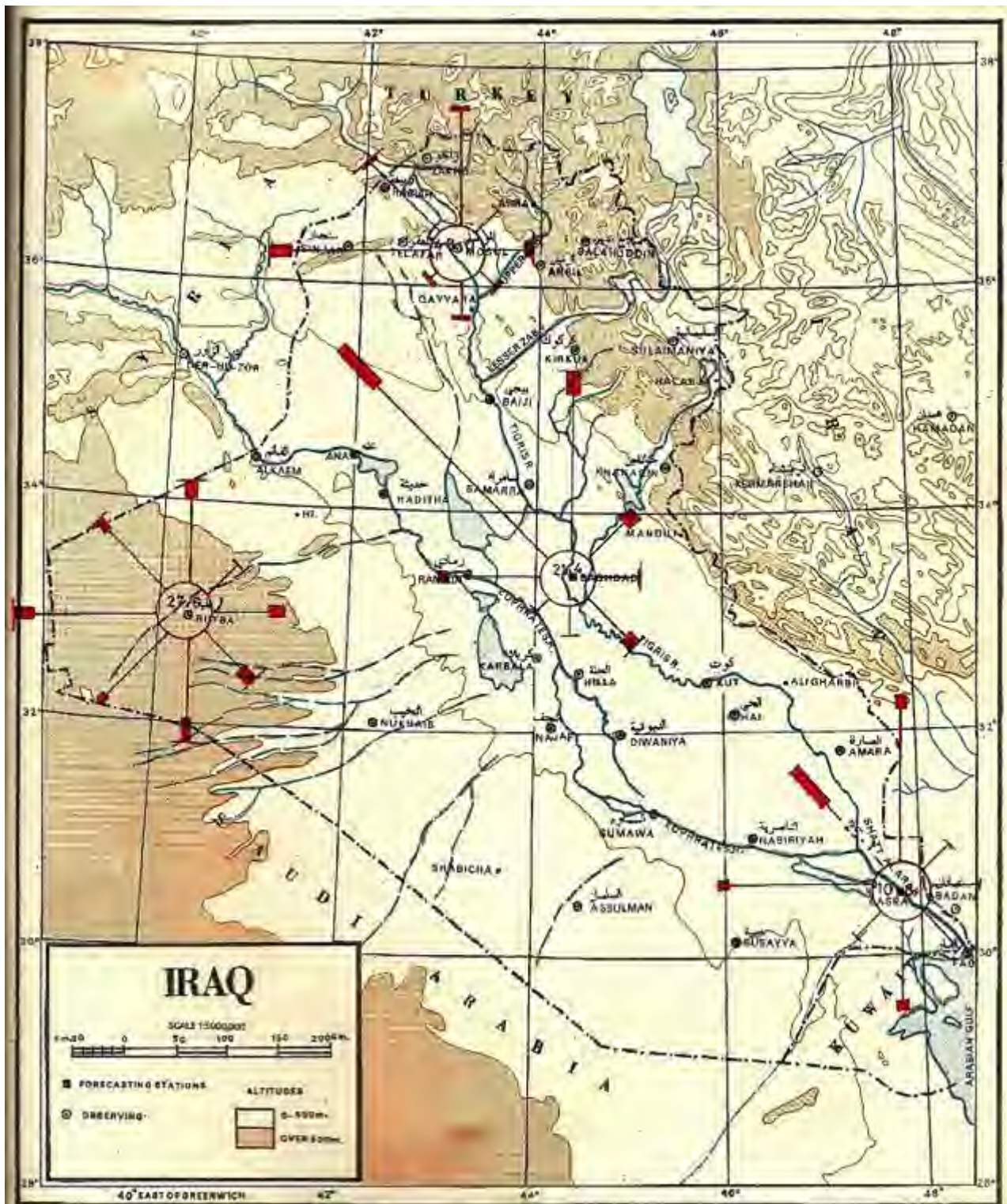
الشكل 2-12: المعدل الشهري لتكرارات الرياح "سرعة واتجاهاً" ضمن الاتجاهات المعينة خلال شهر تشرين الأول [2]
