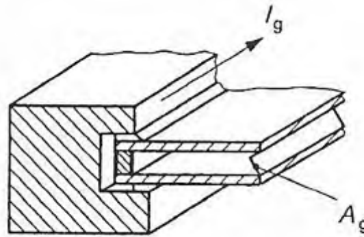
الشكل 2/5-4: توضيح مساحة الزجاج ومحيط التزجيج للنافذة او الباب[4]
