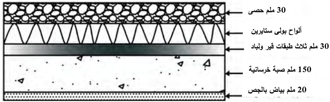
أ- تسطیح باستعمال عازل حراري من نوع ألواح البولي ستايرين الابعاد للمثال فقط
