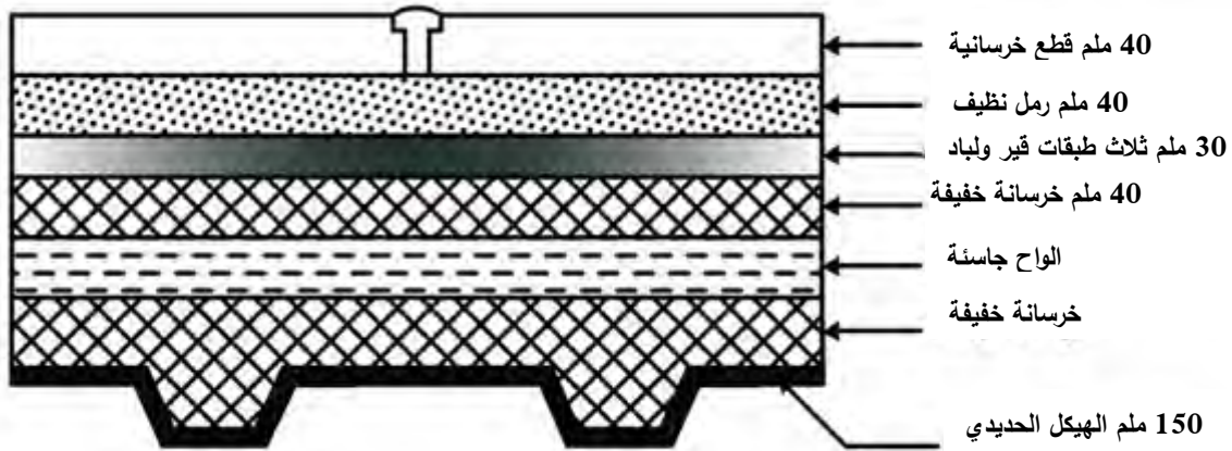
ج- تسطیح باستعمال عازل حراري من نوع ألواح البولي ستايرين في الهياكل الحديدية الابعاد للمثال فقط
