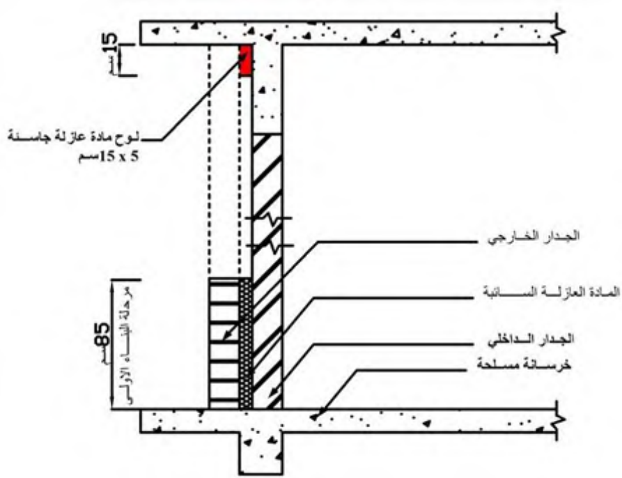
الشكل 7-1/8: طريقة تنفيذ العزل الحراري لجدار مزدوج باستعمال مواد العزل السائبة [5] (يثبت معيق البخار بحسب الفقرة 7-5/4)
