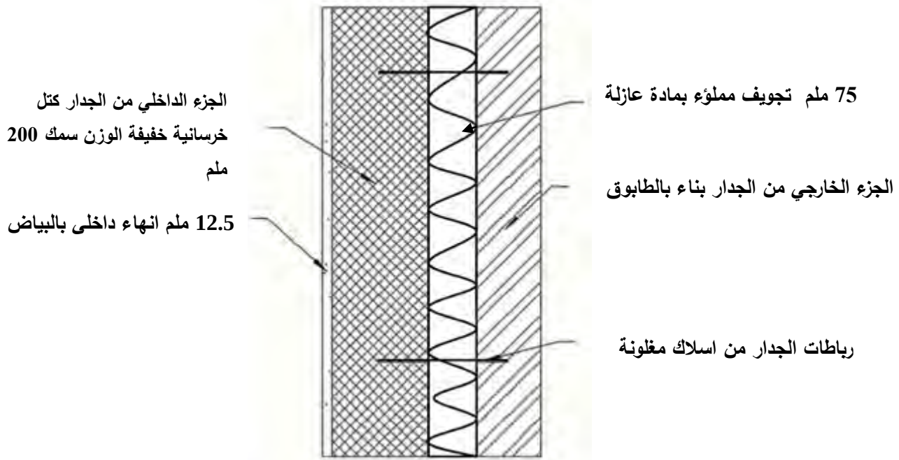
الشكل 3-7: نموذج جدار مزدوج بعزل حراري كلي (الابعاد هي للمثال) [1] ( يثبت معيق البخار بحسب الفقرة 5/4/8-7 )
