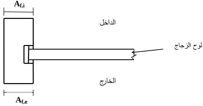
الشكل 4-3/5: مساحة الاسقاط الداخلية والخارجية لإطار النافذة أو الباب [4]
