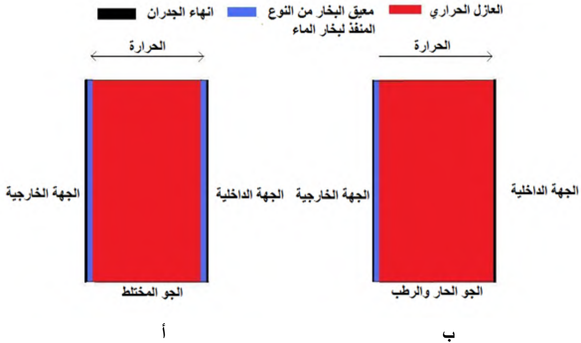
الشكل 5-1/6: أماكن تثبيت معوقات بخار الماء [4]
