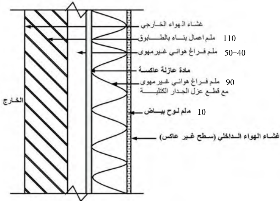
الشكل 7-2/9: مقطع لجدار هيكلي بواجهة من الطابوق (الابعاد هي للمثال) [4] (يثبت معيق البخار بحسب الفقرة 7-5/4/8)
