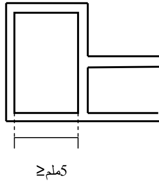
الشكل 4-5/4: تجويف فارغ في مقطع إطار لدائني للنافذة
