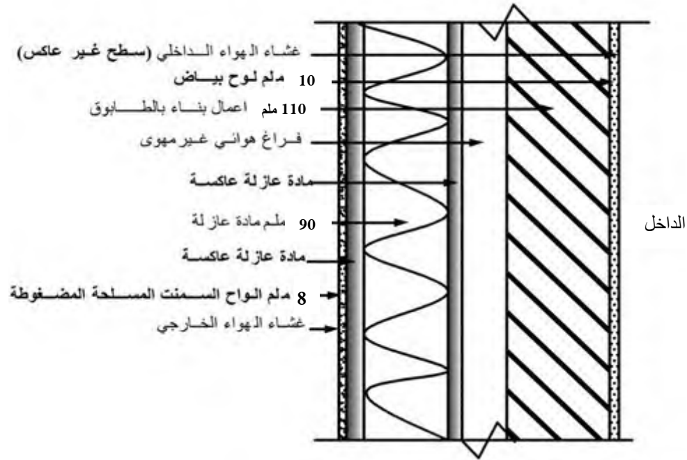
الشكل 7-2/10: مقطع لجدار هيكلي بطبقة داخلية من الطابوق (الابعاد هي للمثال) [4] (يثبت معيق البخار بحسب الفقرة 7-8/5/4)
