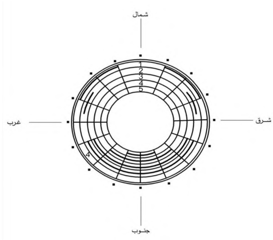
الشكل 2/4-2: توصيات حدود استعمال المصدات الشمسية الثابتة [3]
