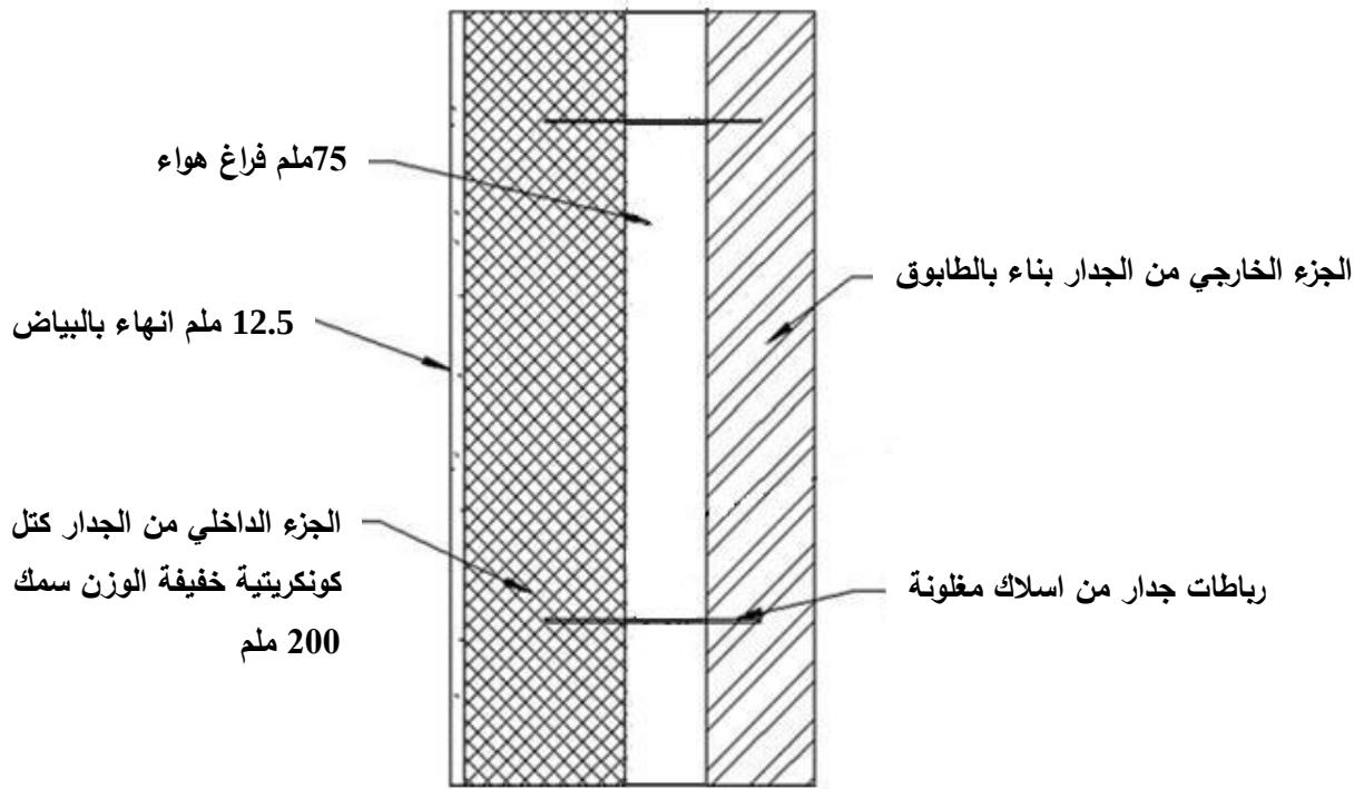
الشكل 7-2/1: نموذج جدار مزدوج بتجويف هوائي لا يحتوي على مادة عازلة (الابعاد هي للمثال) [1] (يثبت معيق البخار بحسب الفقرة 7-5/4/8)
