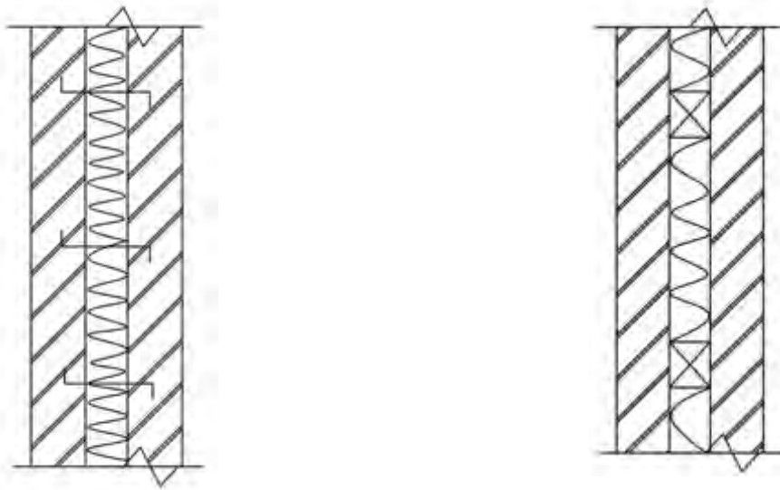
ب- الروابط في الجدران المزدوجة
