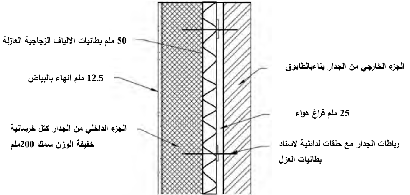
الشكل 7-2/2: نموذج جدار مزدوج بعزل حراري جزئي (الابعاد هي للمثال) [1]
