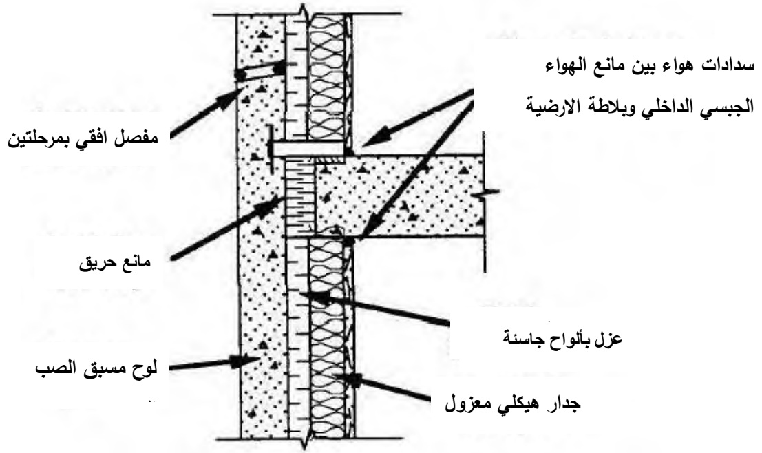
الشكل 7-2/7: جدار مسبق الصب مع عزل جاسيء [2] (يثبت معيق البخار بحسب الفقرة 5/4/8-7)
