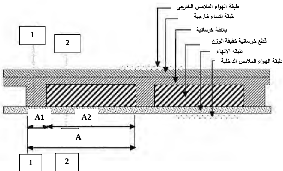
الشكل 10/5-4: تفاصيل عنصر إنشائي غير متجانس التركيب [8]
