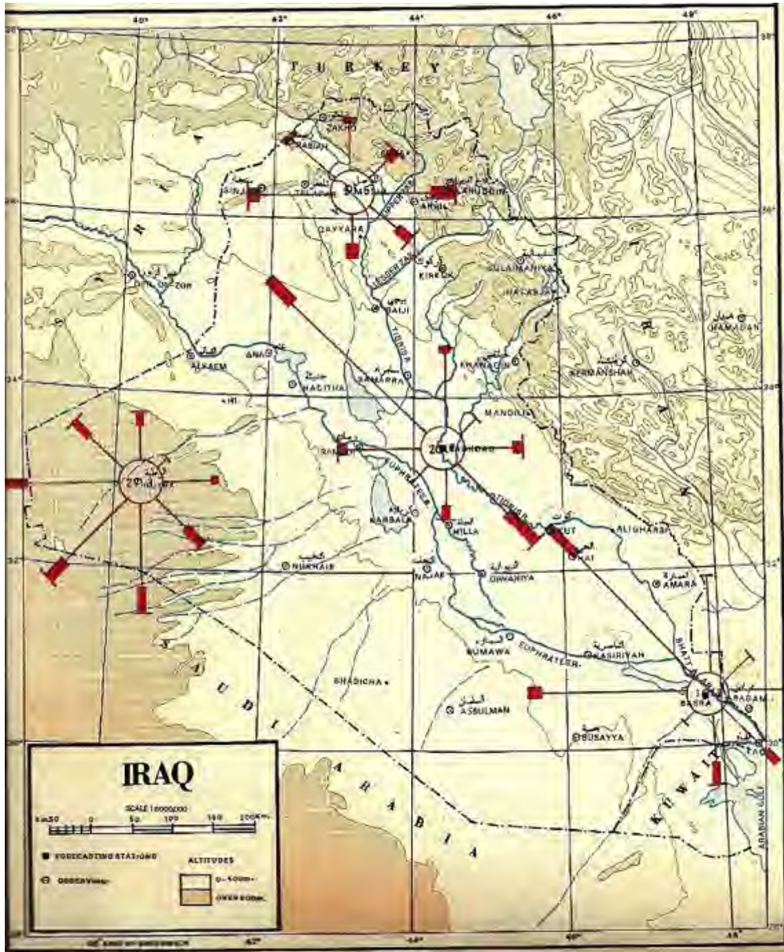
الشكل 2-9: المعدل الشهري لتكرارات الرياح "سرعة واتجاهاً" ضمن الاتجاهات المعينة خلال شهر كانون الثاني [2]
