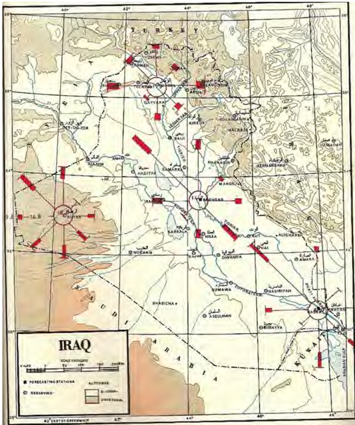
الشكل 2-10: المعدل الشهري لتكرارات الرياح "سرعة واتجاهاً" ضمن الاتجاهات المعينة خلال شهر نيسان [2]
