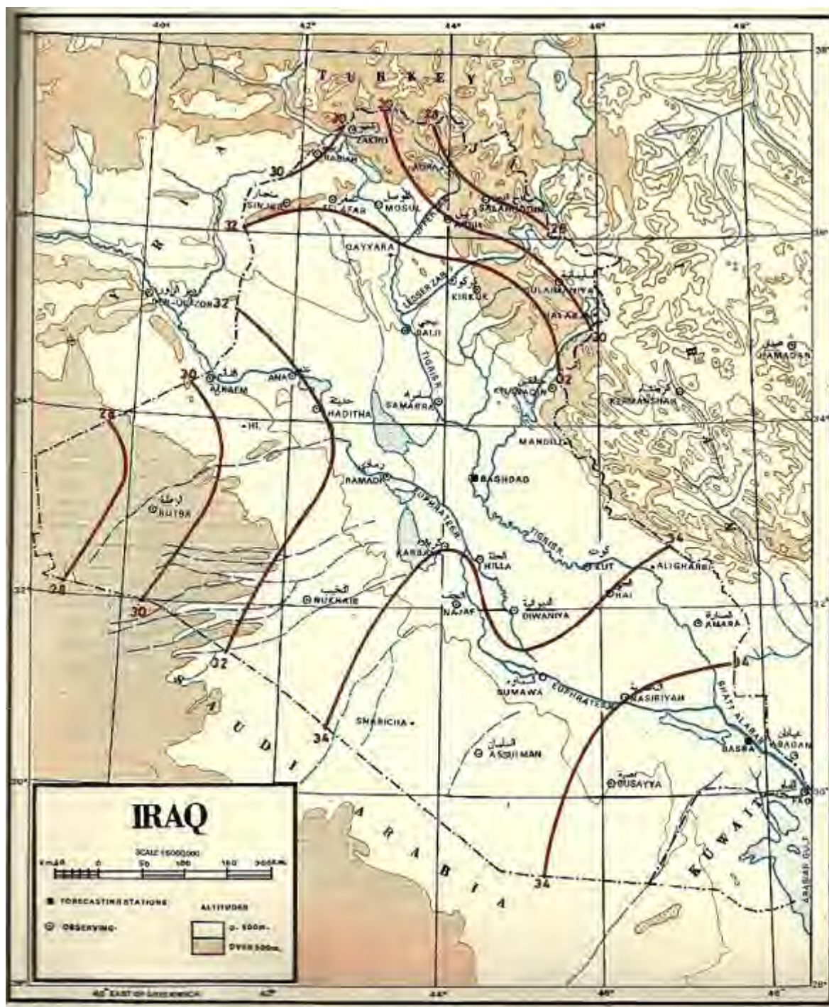
الشكل 2-4: خارطة العراق الكنتورية لمعدل درجات الحرارة لفصل الصيف (مئوي) [2]
