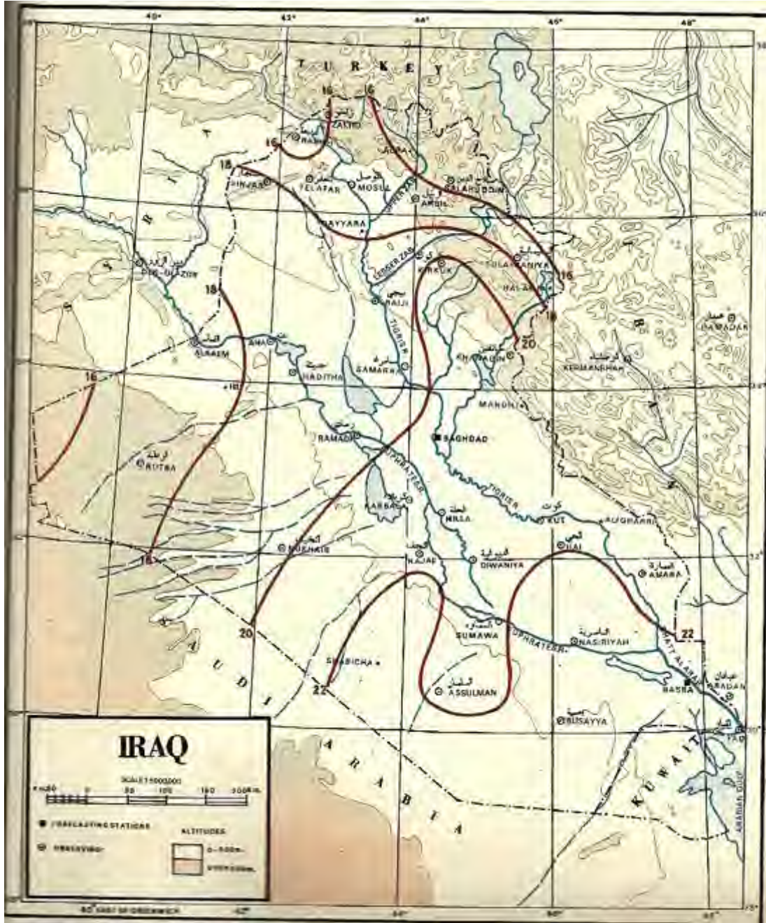
الشكل 2-5/2: خارطة العراق الكنتورية لمعدل درجات الحرارة لفصل الخريف (مئوي) [2]
