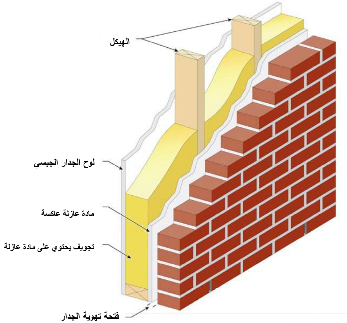
الشكل 8/2-7: جدار هيكل خشبي بواجهة من الطابوق الطيني [3] (يثبت معيق البخار بحسب الفقرة 5/4/8-7)
