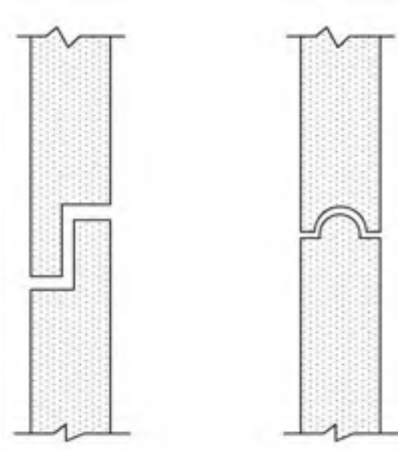
الشكل 7-4/8: أنواع المفاصل للألواح العازلة الجاسئة المستعملة في الجدران [5]
