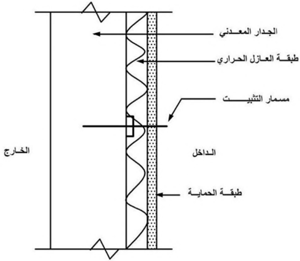
الشكل 3/8-7: طريقة العزل الحراري لجدار منفرد معدني باستعمال المواد العازلة شبه الجاسئة [5] (يثبت معيق البخار بحسب الفقرة 5/4/8-7)
