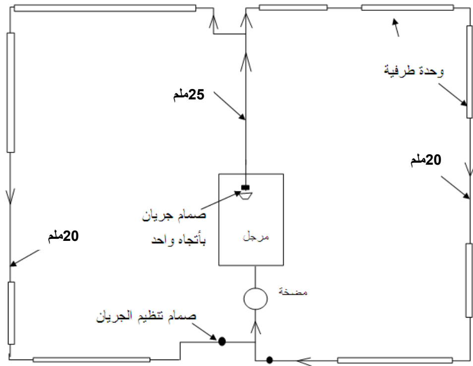
الشكل 3-1: منظومة ربط شبكة أنابيب متوالية
