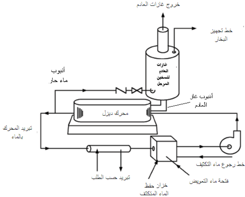
الشكل 3-3 : مرجل الحرارة الفائضة
