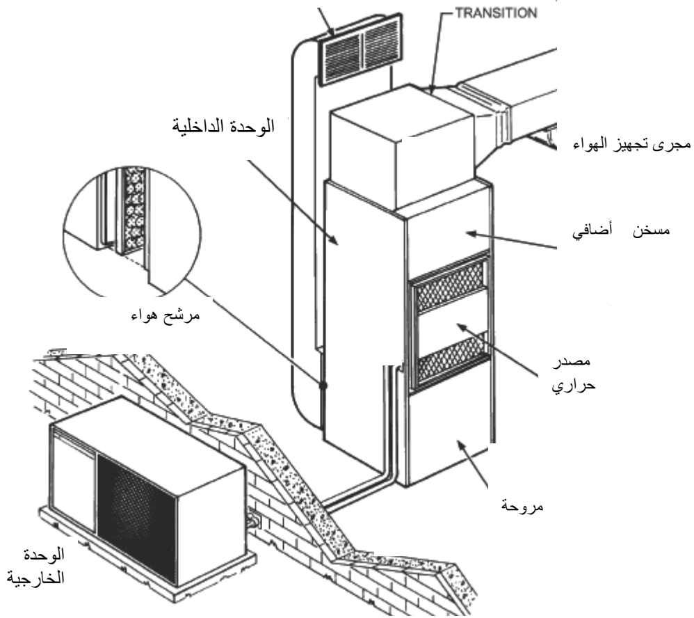
الشكل 3-1 : منظومة تدفئة منزلية مجمعة نموذجية
