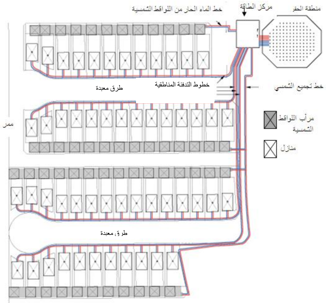
الشكل 3-2 : منظومة تدفئة مناطقية باعتماد الطاقة الشمسية
