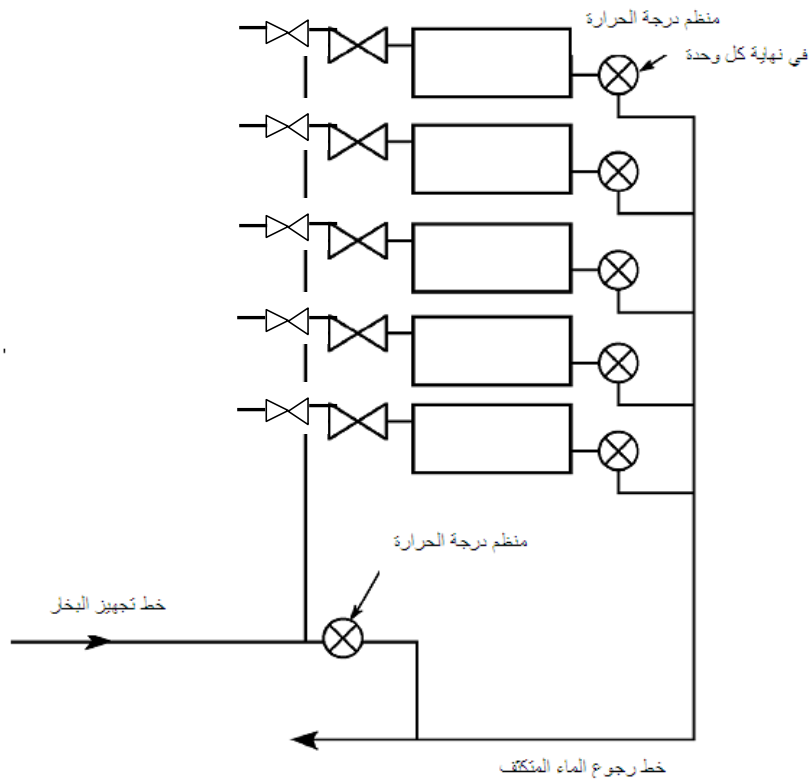
الشكل 3-2/4 : منظومة التسخين ذات الأنبوبين
