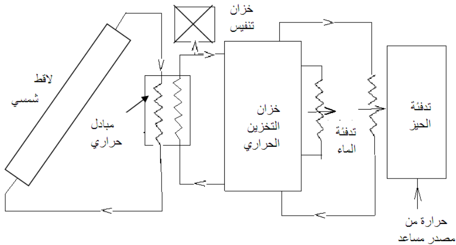
الشكل 3-1/4 : منظومة شمسية لتسخين المنازل
