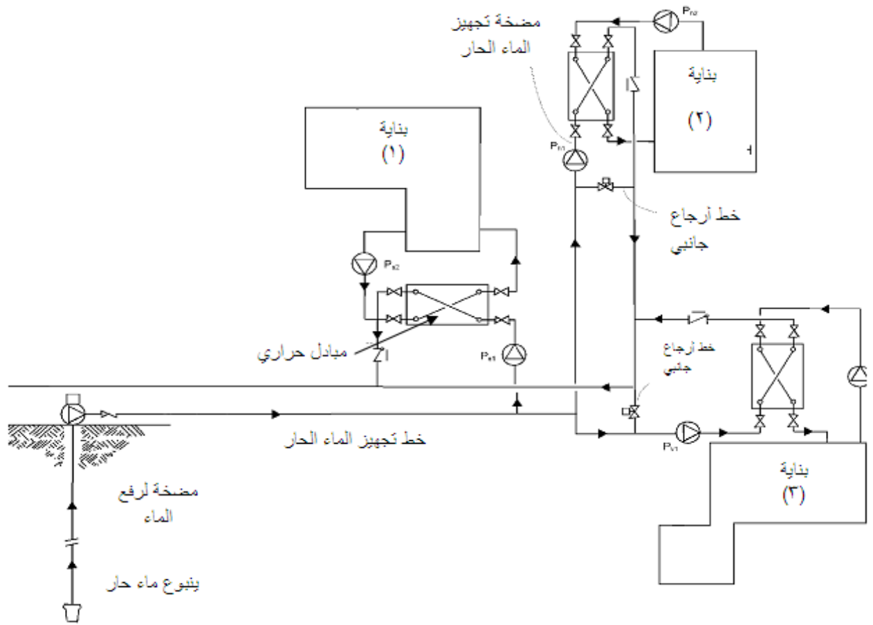
الشكل 3-5 : منظومة تدفئة مناطقية باعتماد طاقة باطن الأرض
