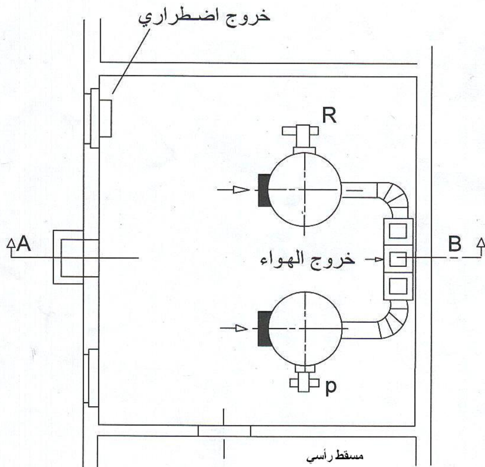
الشكل 5-2/1: تهوية غرفة التسخين بالوقود السائل
