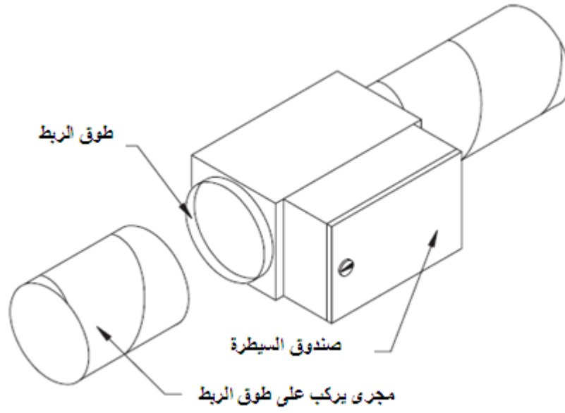
الشكل 3-6/2 : مسخن لمجري مدور المقطع
