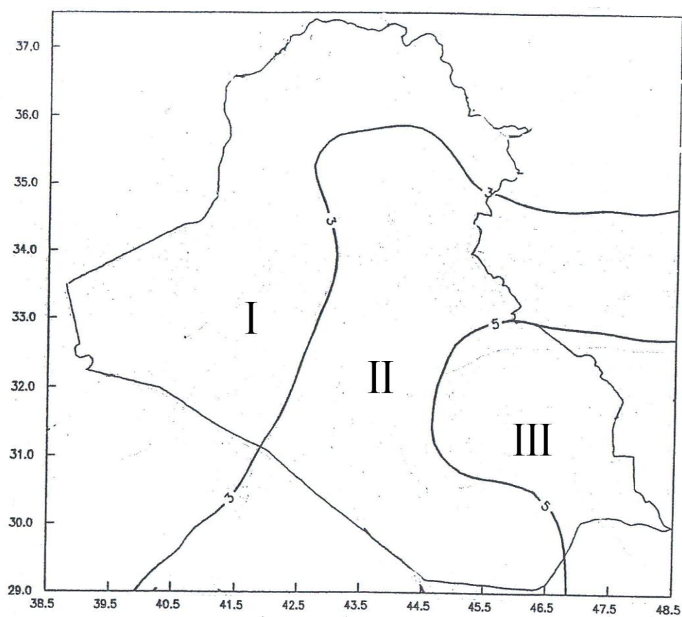
الشكل 1-3/6 : تقسيم العراق الى ثلاث مناطق حرارية
