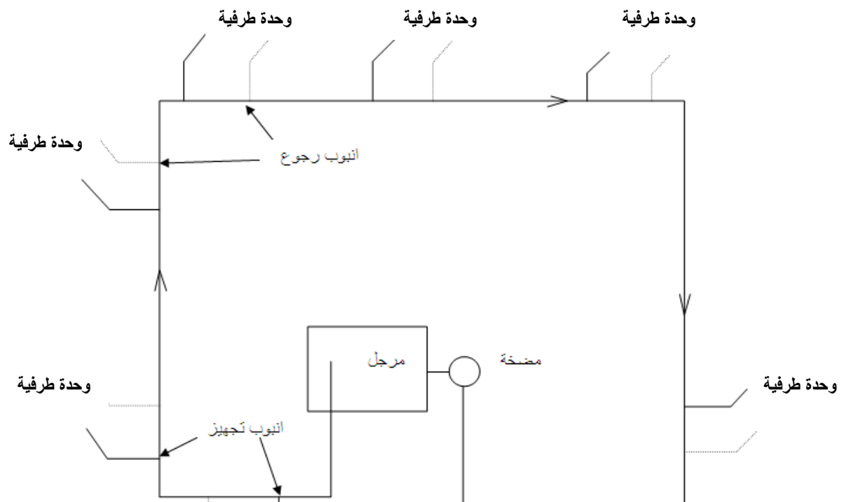
الشكل 3-2: منظومة ربط الأنابيب الواحد
