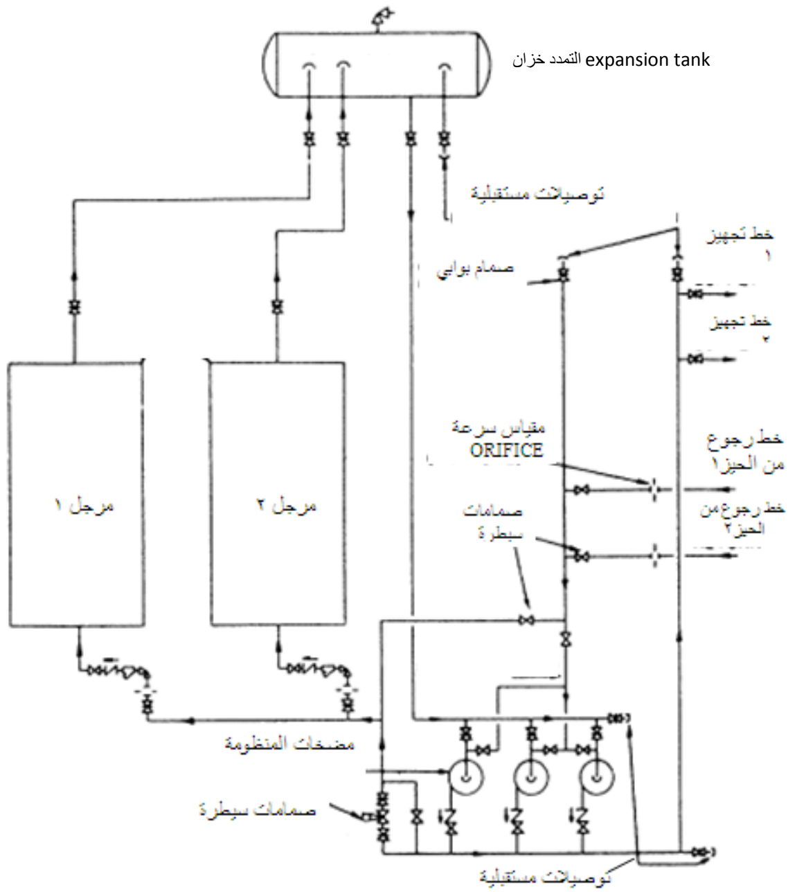
الشكل 3-5: مجموعة الضخ المنفردة لمنظومة ماء حار عالية درجة الحرارة
