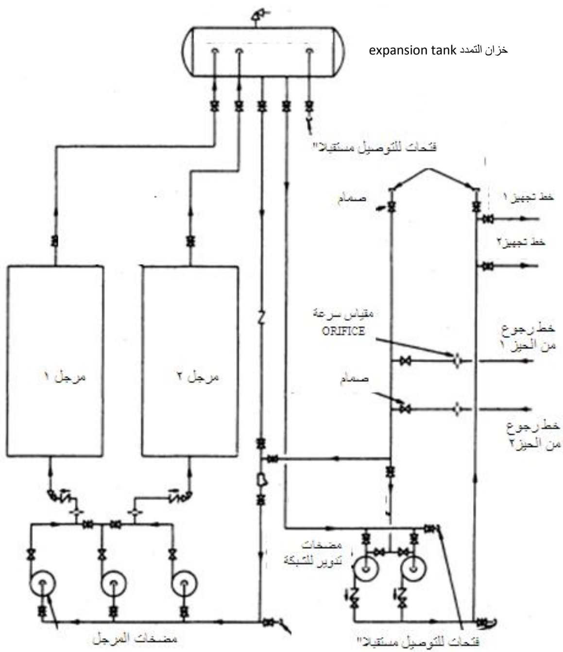
الشكل 3-3/6 : مجموعة الضخ الثنائية لمنظومة ماء حار عالية درجة الحرارة
