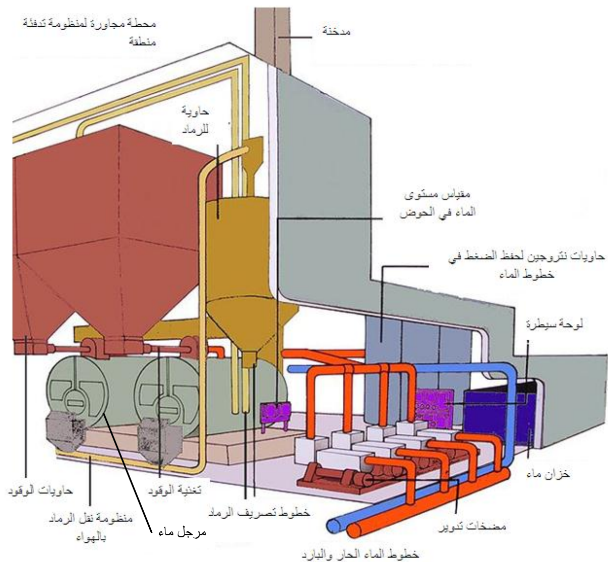
الشكل 3-1 : منظومة تدفئة مناطقية من محطة توليد الكهرباء
