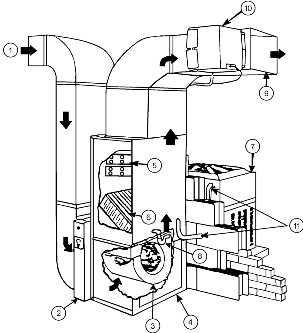
الشكل 3-2 : منظومة مضخة حرارية منزلية نموذجية
