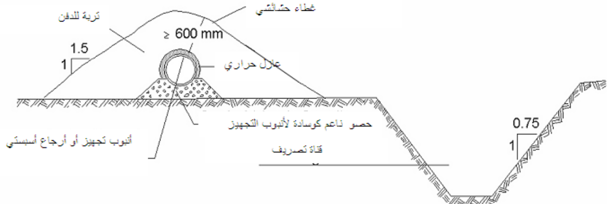
الشكل 3-5 : عزل ودفن أنابيب منظومة التدفئة المناطقية
