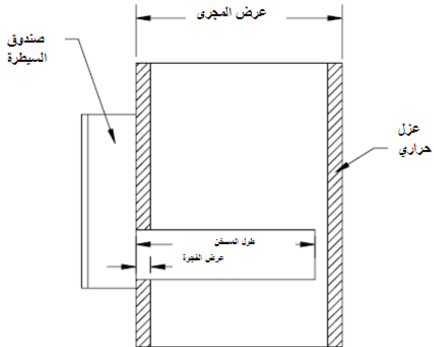
الشكل 3-6/3 : مسخن لمجري معزول
