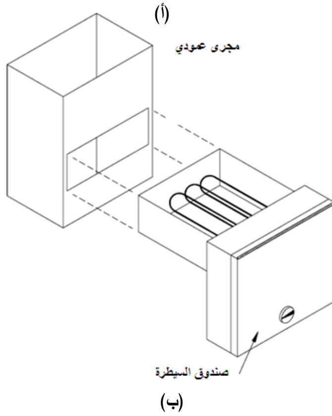
الشكل 3-1/6 : مسخن لمجري هواء (أ) أفقي (ب) عمودي
