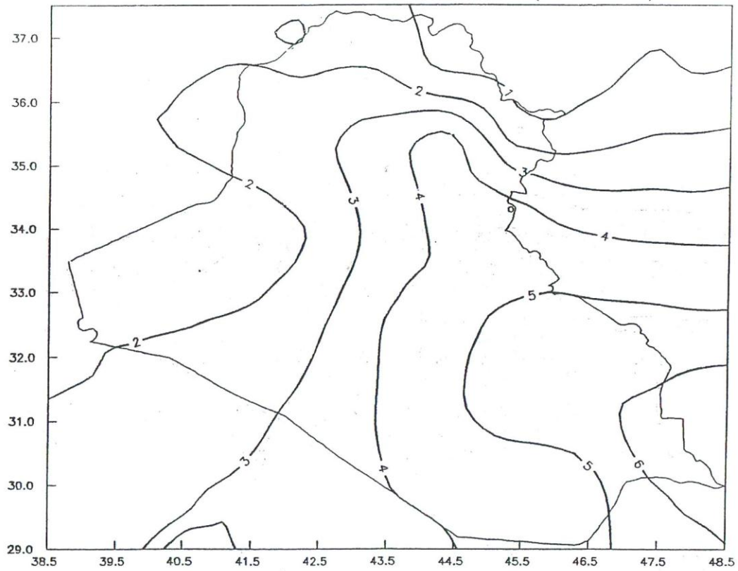
الشكل 1-4 : المعدلات الشهرية لدرجة الحرارة الصغرى بالدرجات السيلزية (كانون الثاني)
