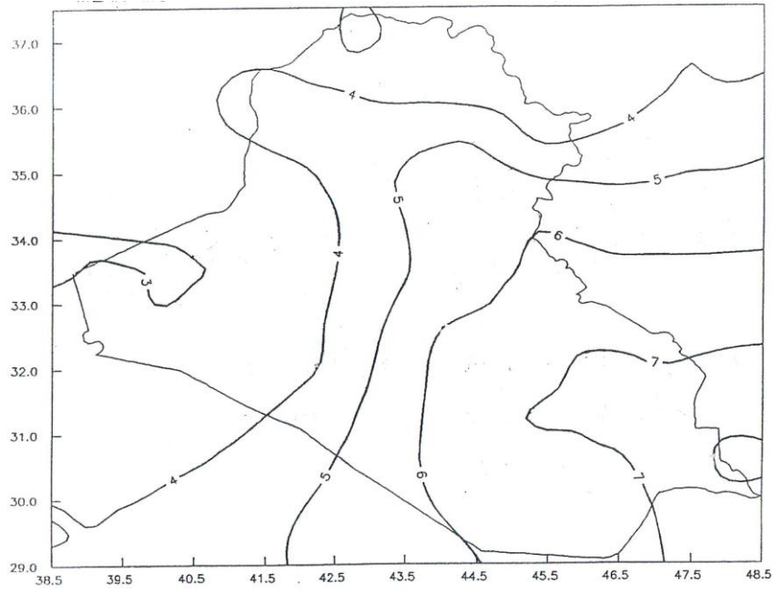
الشكل 1-3 : المعدلات الشهرية لدرجة الحرارة الصغرى بالدرجات السيلزية (كانون الأول)
