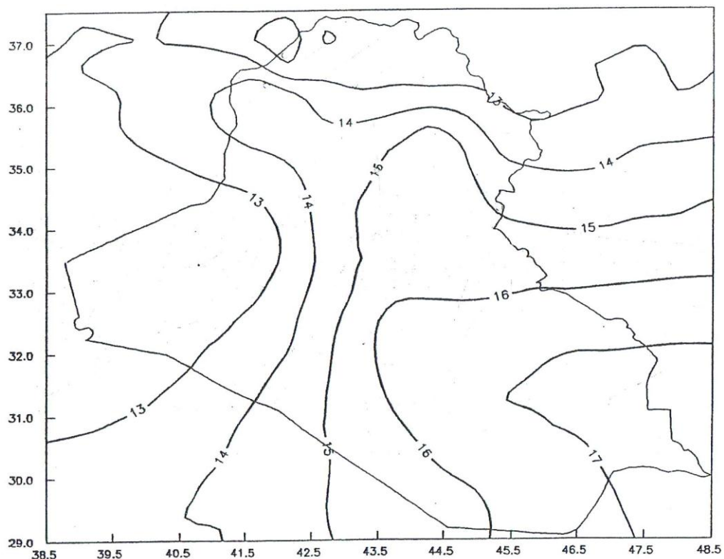
الشكل 1-2/3 : المعدلات السنوية لدرجة الحرارة الصغرى بالدرجات السيلزية
