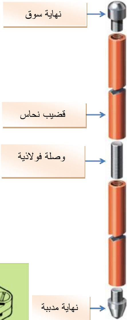
تفاصيل قضيب التأريض
