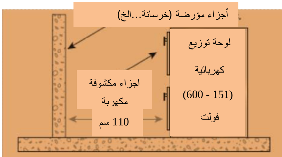
الحالة الثانية: الفولتيات (600-151) فولت أقل فضاء هو \leq 110 سم
