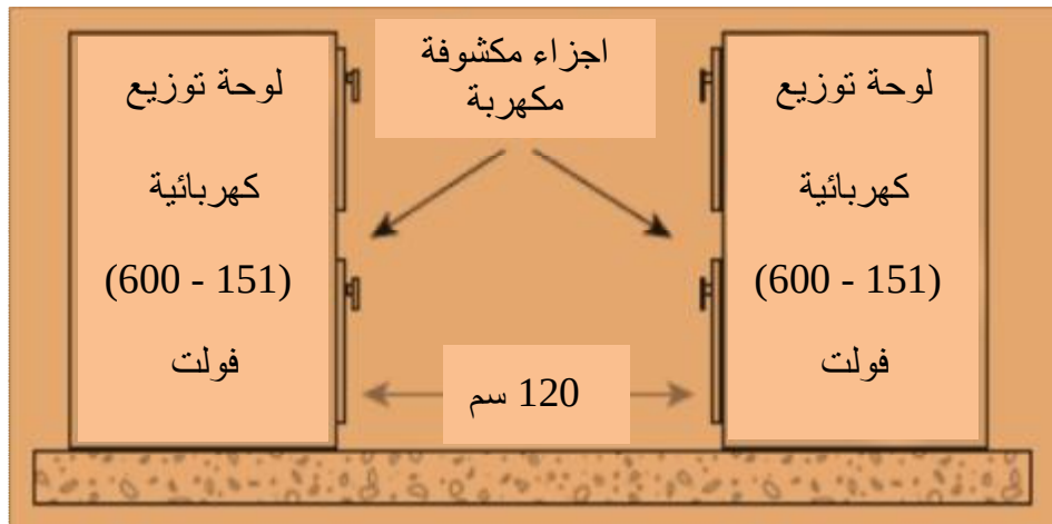
الحالة الثالثة: الفولتيات (600 - 151) فولت أقل فضاء هو \leq 120 سم
