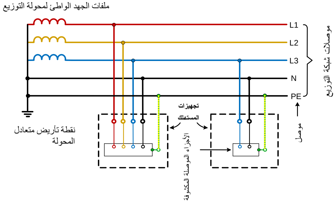
نظام تأريض من النوع TN-S
