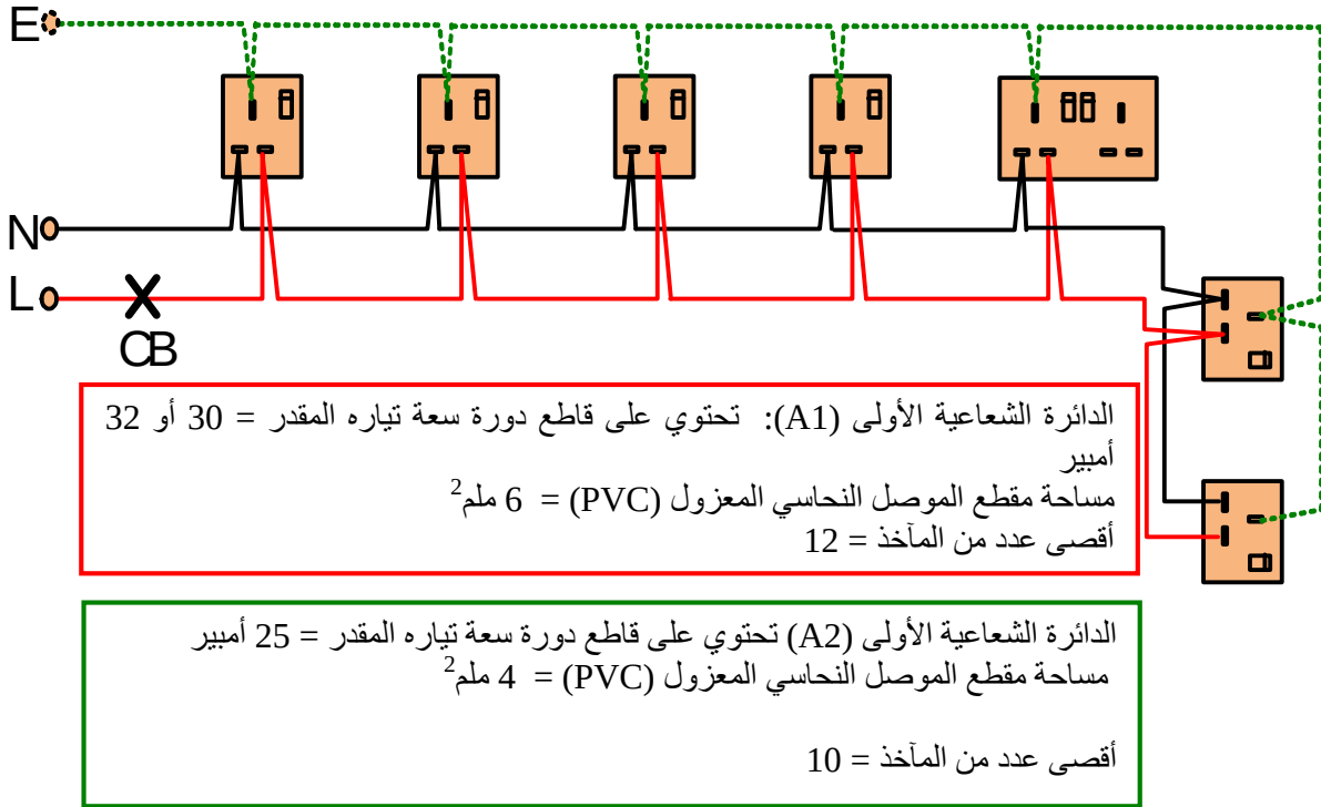
الشكل 2/2-3: الدائرة الشعاعية (Radial Circuit)
