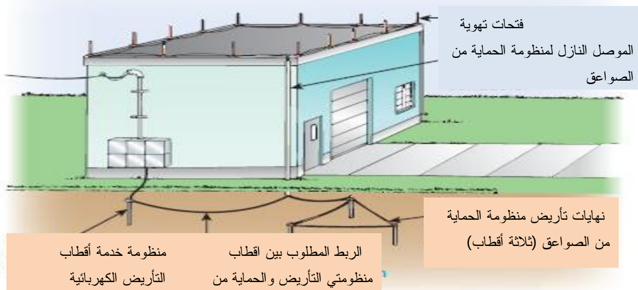
الشكل 9-1/8: ربط نظامي التأريض لممانعة الصواعق والتأسيسات الكهربائية للمباني
