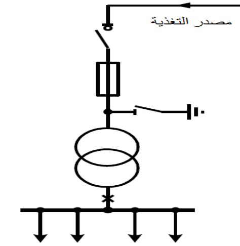
الشكل 1/5-7: طريقة التجهيز المنفرد
