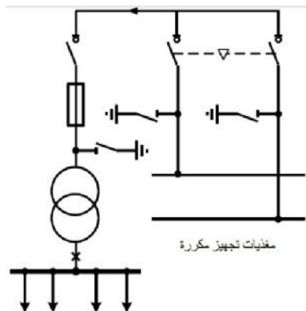
الشكل 3/5-7: طريقة التجهيز المزدوج
