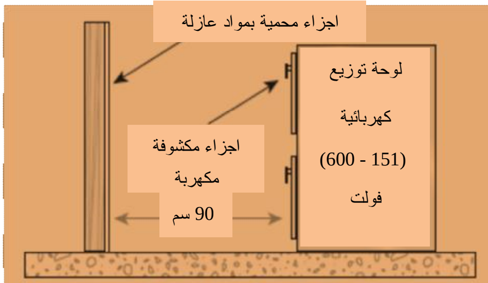
الحالة الأولى: الفولتيات (600-151) فولت أقل فضاء هو \leq 90 سم
