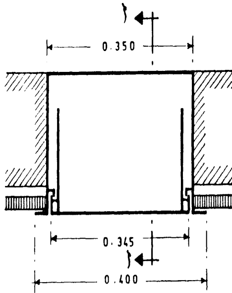
الشكل 7-1/6: قادوس أنموذجي من المعدن (كودة النفايات الاردنية، 2003)
