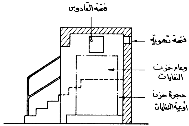
مقطع أ-أ
