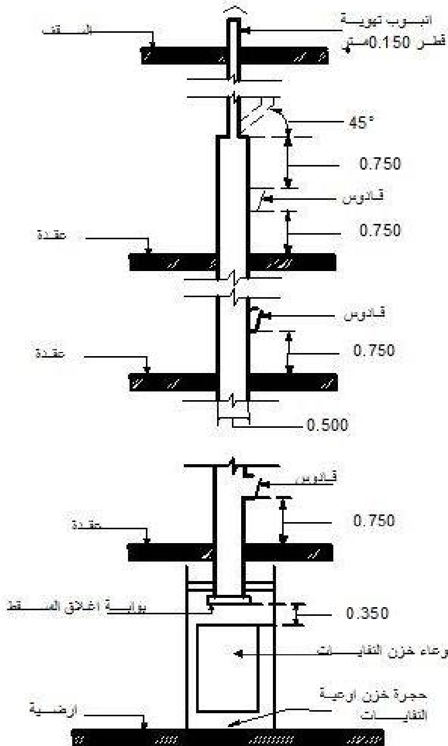
الشكل 7-1/3: مقطع أنموذجي لمسقط النفايات والقواويس المتصلة به وحجرة خزن أوعية النفايات (كودة النفايات الاردنية، 2003)
