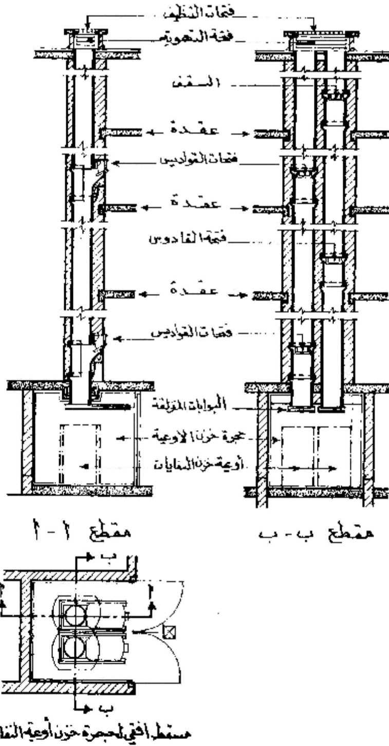
الشكل 7-2/5: شكل أنموذجي يبين تركيب مسطحي نفايات مشتركين بحجرة واحدة في الابنية متعددة الطوابق (كودة النفايات الاردنية، 2003)
