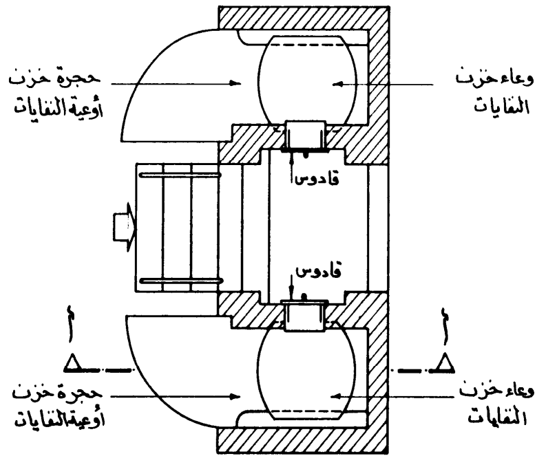
المقطع الأفقي
